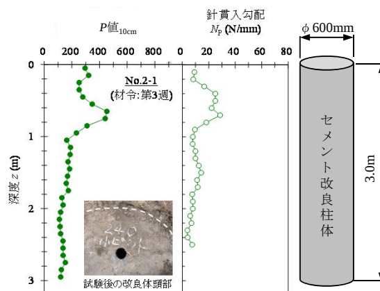
図-7.セメント改良体品質確認調査結果例 (小型RPD+小型ビット)
