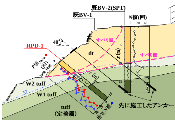
図-4.グラウンドアンカーの削孔管理適用例(大型RPD+大型ビット)
